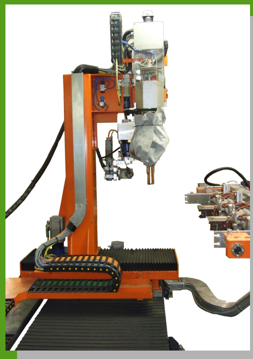
AFFILATURA ELETTRODI IN AUTOMATICO FINO A 6 ASSI CNC TAVOLA ROTANTE
