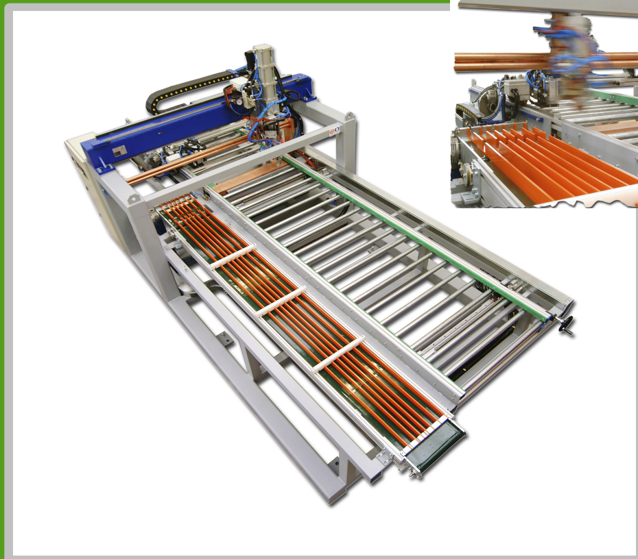
ISOLA ROBOTIZZATA AD ASSE CARTESIANO SETTORE AUTOMOBILISTICO
